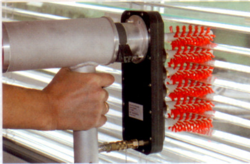
Spezialbürsten schonen die hochreflektierende Oberflächen-Beschichtung einer TLT-Jalousie
